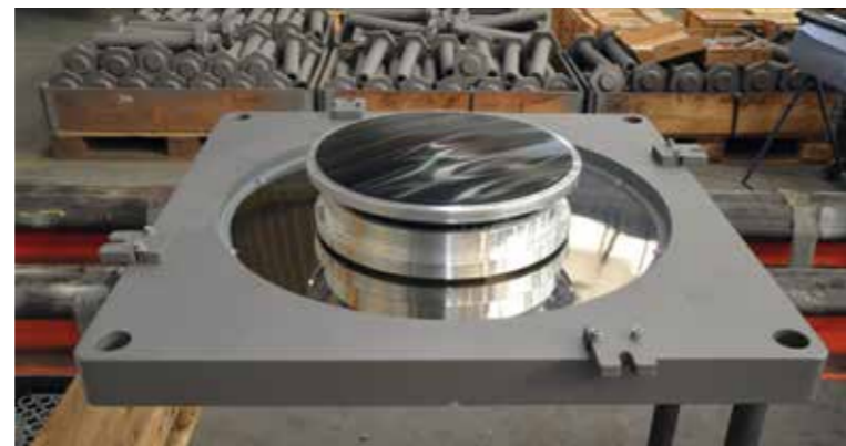
Untere Gleitfläche mit gelenkigem Gleiter
